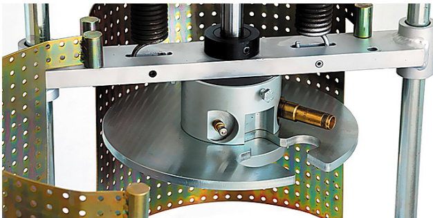
Hidropnömatik Pompa Hydropneumatic Pump
